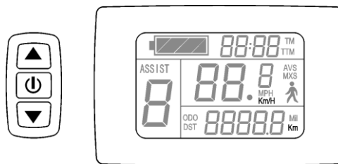
公制/英制单位设置界面
