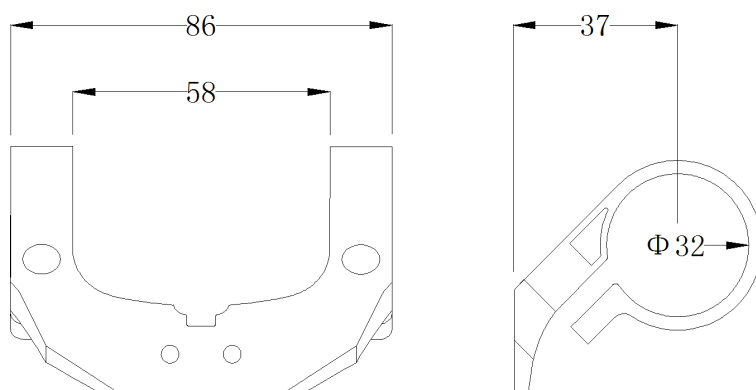
双支架安装尺寸
