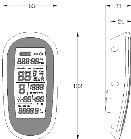
仪表主体外形尺寸
