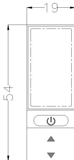
仪表主体外形尺寸
